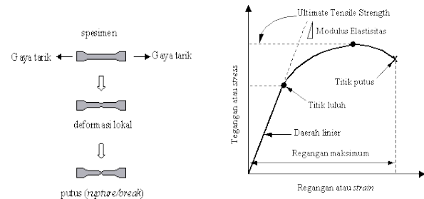
Gambar 5. Diagram Tegangan Renggang
