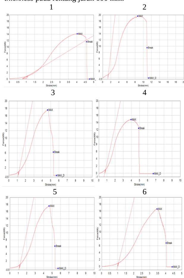
Gambar 6 Kurva Uji Tarik
