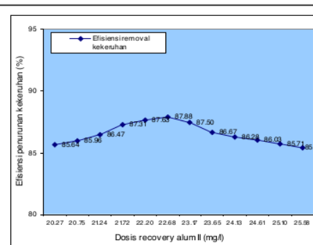
Gambar 8b Hubungan antara Dosis Recovery Alum II terhadap Efisiensi Penurunan Kekeruhan dengan Kekeruhan Awal 15,6 NTU
