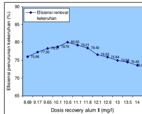
Gambar 7b Hubungan antara Dosis Recovery Alum II terhadap Efisiensi Penurunan Kekeruhan dengan Kekeruhan Awal 8,9 NTU
