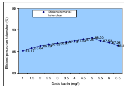
Gambar 9b Hubungan antara Dosis Alum+Kaolin terhadap Efisiensi Penurunan Kekeruhan dengan Kekeruhan Awal 8.9 NTU
