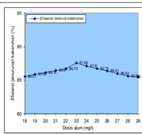
Gambar 4b Hubungan antara Dosis Aluminium Sulfat terhadap Efisiensi Penurunan Kekeruhan dengan Kekeruhan Awal 15,6 NTU
