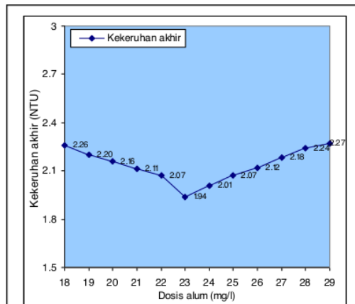
Gambar 4a Hubungan antara Dosis Aluminium Sulfat terhadap Kekeruhan Akhir dengan Kekeruhan Awal 15,6 NTU
