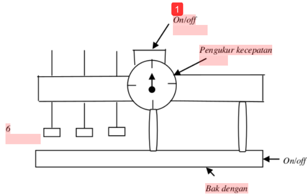
Gambar 1 Alat Jar tes untuk Koagulasi-Flokulasi (Phips dan Bird)
