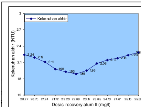
Gambar 8a Hubungan antara Dosis Recovery Alum II terhadap Kekeruhan Akhir dengan Kekeruhan Awal 15,6 NTU
