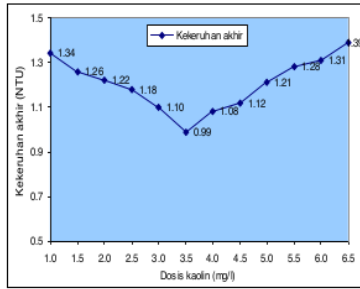
Gambar 13a Hubungan antara Dosis Recovery Alum II+Kaolin terhadap Kekeruhan Akhir dengan Kekeruhan Awal 8,9 NTU
