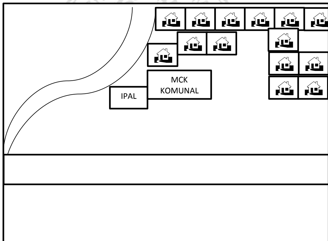
Gambar 6 : Denah MCK Komunal Dan IPAL Desa Pecoro
