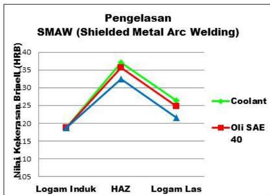
Gambar 2. Grafik Nilai Kekerasan pada Pengelasan SMAW ( Shielded Metal Arc Welding )
