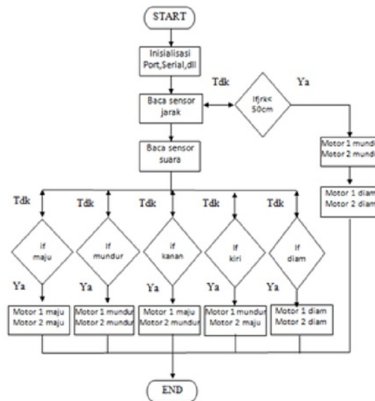
Gambar 7. Flowchart Kontrol Utama Alat
