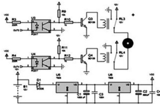
Gambar 6. Diagram Skematik Keseluruhan Sistem
