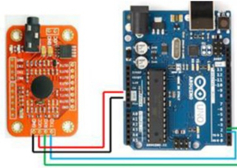
Gambar 1. Menghubungkan Modul VR3 dan Arduino Uno R3
