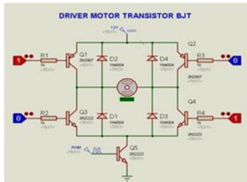
Gambar 2. Motor Driver dengan Transistor
