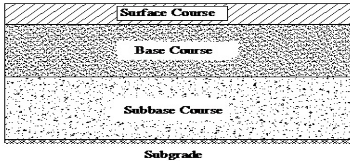
Gambar 2.1. Susunan Lapisan Perkerasan Jalan
