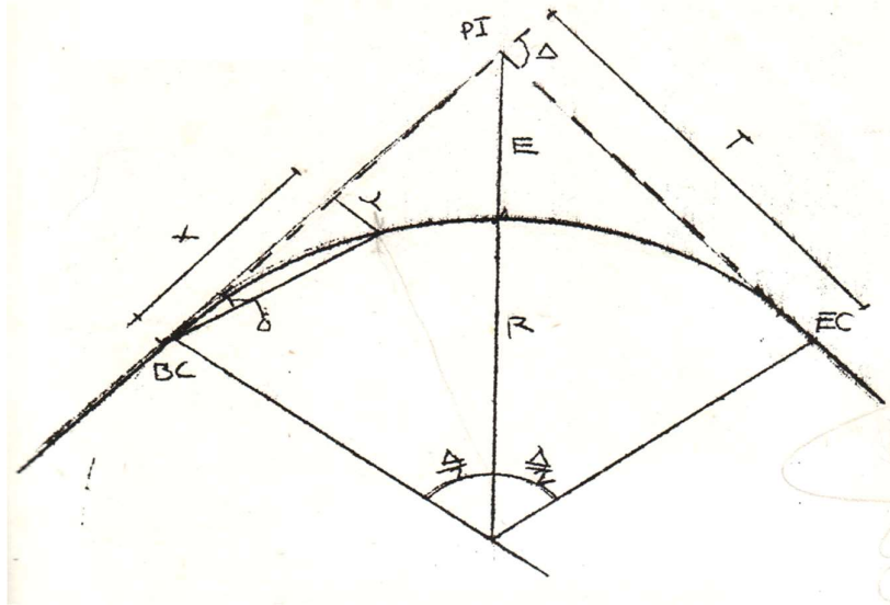
Gambar 2.1 Tikungan jenis full circle
