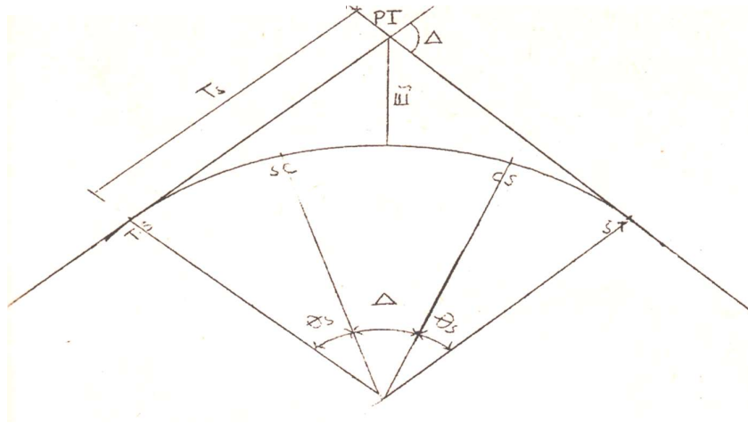
Gambar 2.2 Tikungan jenis spiral-circle-spiral
