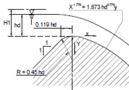
Gambar. Perencanaan mercu Ogee
