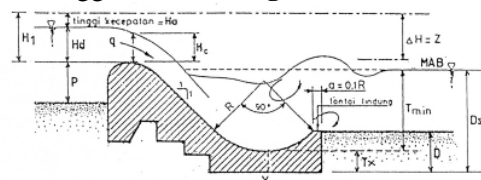
Gambar. Peredam energi tipe bak tenggelam
