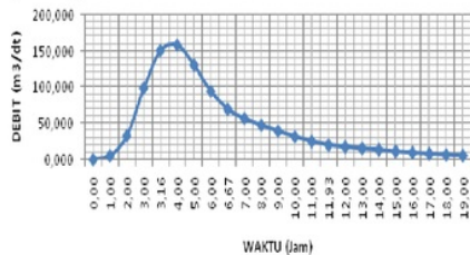
Gambar 9. Hidrograf Banjir Nakayasu pada tanggal 1 Januari 2006
