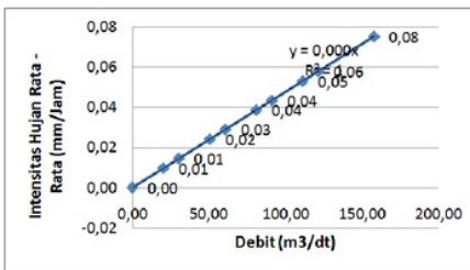
Gambar 12. Grafik hubungan antara intensitas hujan rata – rata dan debit banjir
