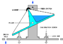
Gambar 2. Sistem penangkap hujan tipe tipping bucket
