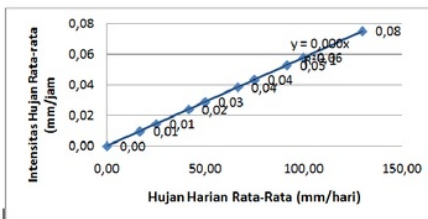
Gambar 13. Grafik hubungan antara intensitas hujan harian rata – rata dan hujan harian rata – rata
