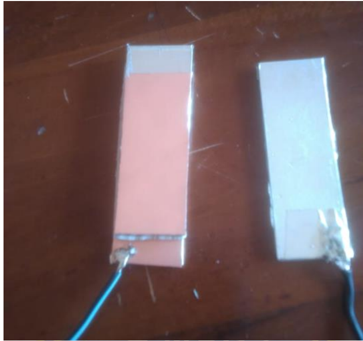
Gambar L-2.9 Perangkaian Elektroda
