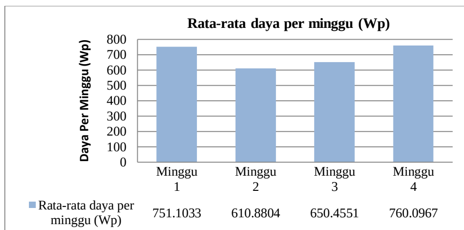
Gambar 6. Grafik Daya Panel Surya Selama 4 Minggu
