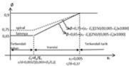
Gambar 3. Nilai faktor reduksi \phi (Priyono,P.(2017))
