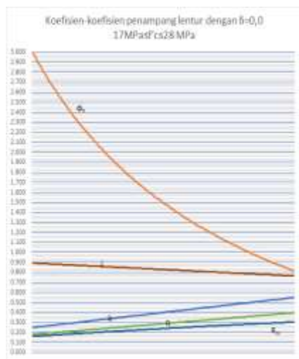
Gambar 5. Grafik nilai koefisien-koefisien penampang lentur dengan \delta=0,0 .
