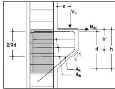
Gambar 7. Konsol Pendek
