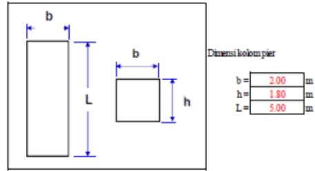
Gambar 8. Dimensi Kolom Pier Sta. 0+400
