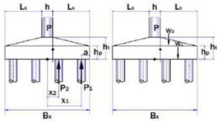
Gambar 9. Pile Cap Arah-x
