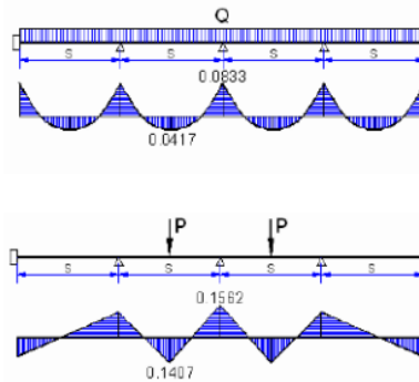
Gambar 17. Konfigurasi Pembebanan dengan Tumpuan Monolit (s = 6 meter)
