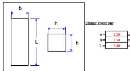
Gambar 13. Dimensi Kolom Pier Sta. 2+30 (1500 x 1200)
