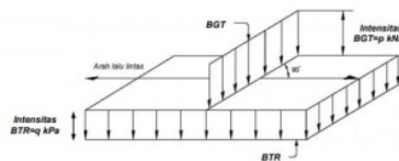
Gambar 3. Beban Lajur D, Konfigurasi BGT dan BTR (SNI 1725 Tahun 2016)
