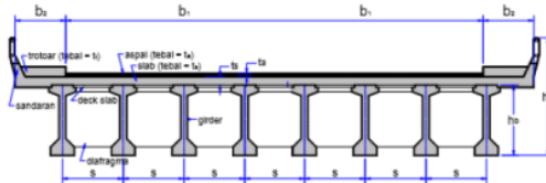
Gambar 18. Potongan Melintang Pelat Lantai Jembatan
