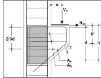
Gambar 7. Konsol Pendek
