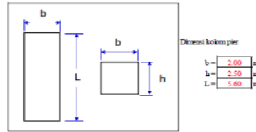
Gambar 14. Dimensi Kolom Pier Sta. 0+750 bentang 30 meter
