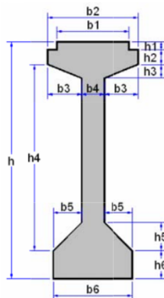
Gambar 2 Dimensi penampang gelagar I
