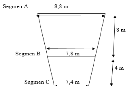
Gambar 3.1 Segmen Plat
