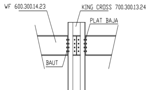
Gambar 3.4 Sambungan Kolom – Balok tampak Depan Samping
