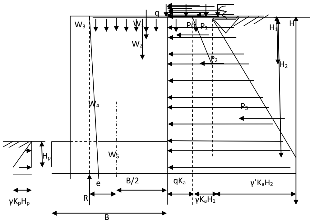
Gambar 5. Tembok penahan tanah dengan distribusi beban
