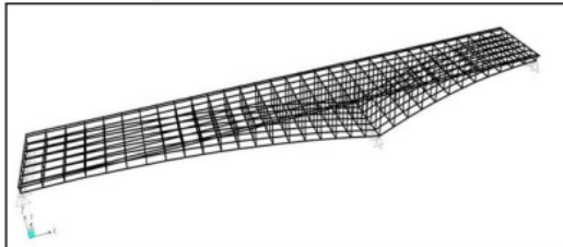
Gambar 8. Gambar SAP2000 Tampak 3-d
