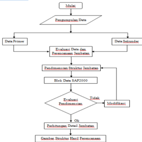
Gambar 3.1 Diagram alir perencanaan jembatan.
